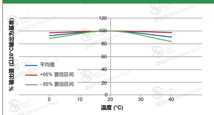
盛密科技4SM CL2-5传感器温度性能
